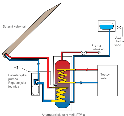
Schema solarnog kolektorskog sustava
