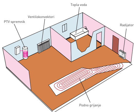
Shema sustava s geotermalnom dizalicom topline
