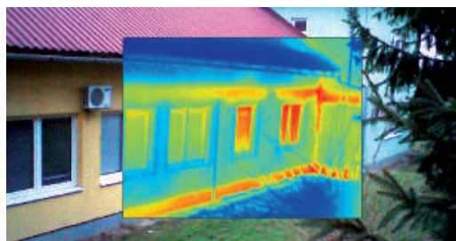
Toplinski nezadovoljavajuće izolirana zgrada
