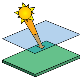
Efekt staklenika
